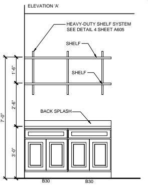
E INTERIOR ELEVATION SCALE: 1/2" = 1'-0"
