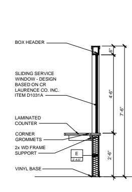
5 INTERIOR ELEVATION SCALE: 1/2" = 1'-0"
