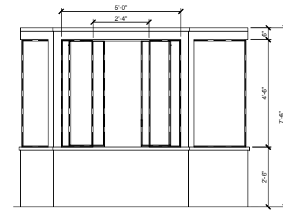
7 INTERIOR ELEVATION SCALE: 1/2" = 1'-0"
